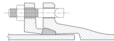
Junta Mecánica (3"-24")
